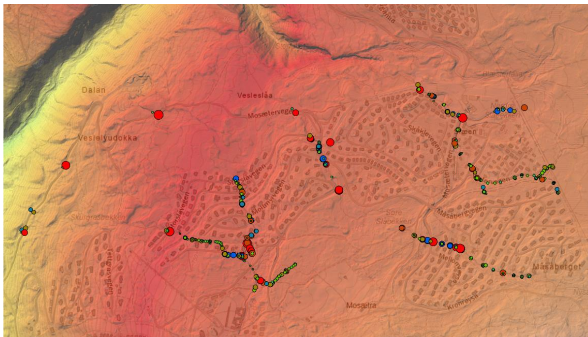
Figur 4-10: Innmålinger foretatt 26.06.2022, større symbol viser større differanse mellom innmålingen og terrenngmodellen. Ved rød farge i punktene er terrenngmodellen høyere enn innmålt punkt, og ved blå farge er den lavere. Bakgrunnsfarge er definert av høyden på terrenngmodellen. Gjennomsnittlig avvik ligger omtrent på 40 cm, men de aller fleste punktene ligger innenfor en forskjell på +/- 15 cm.
