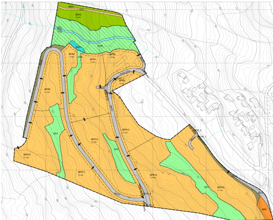
Plankart Kringelåslia nedre FB12 og FB13
