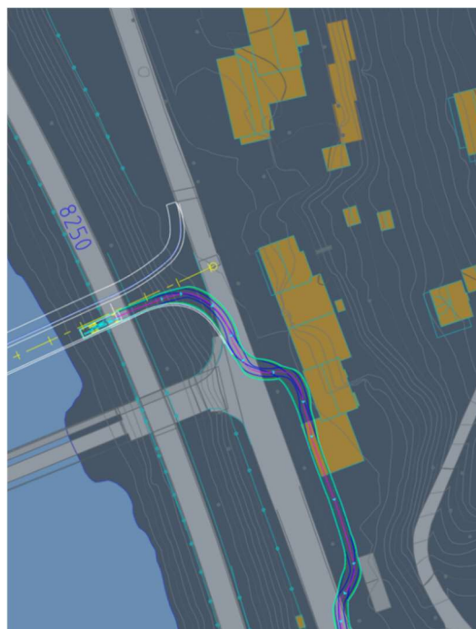
Figur 1-8 Springkurver for lastebil, innkjøring til Circle K fra bru og videre sørover. Bilister må først kjøre ut på Kongsvegen for deretter å kjøre av inn mot Circle K.
