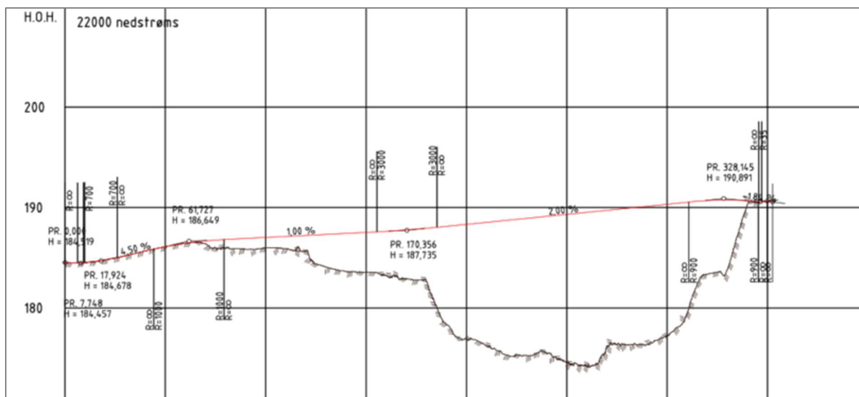
Figur 1-3 Lengdeprofil alternativ 2 nedstrøms dagens bru. Den røde linja viser stigningsforhold på brua og at høybrekket er over kulverten for E6. En stigning på 1-2 % på brua framstår som om den er horisontal.
