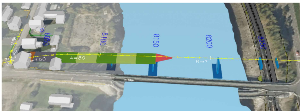
Figur 1-7 Prinsipp for framføring (lansering) av bru alternativ 1 - Bru oppstrøms dagens bru. Det etableres byggegrop i deler av svart markering, ca. 1,5 meter under dagens terreng.
